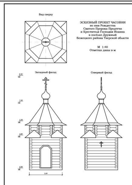
Эскизный проект часовни на святом источнике Иоанна Крестителя в пос. Дружный.
